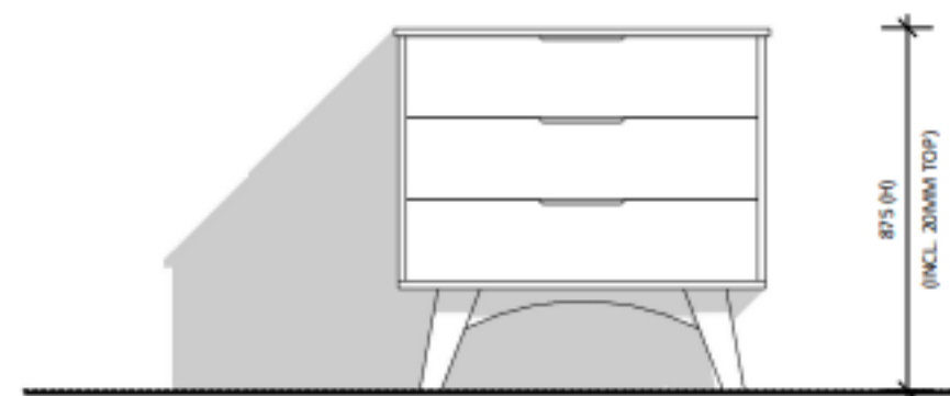
E1 FRONT 01 scale 1:20
